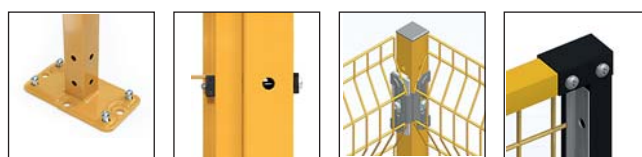
Sposoby montażu elementów wygradzeń
