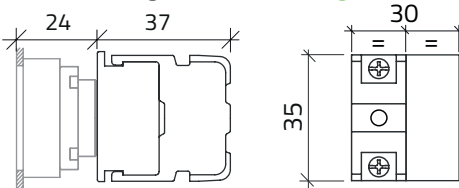
1 NO con flangia / 1NO with flange
