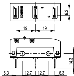
Pionowe styki H
