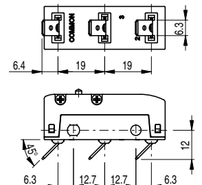
styki G , skierowane w lewo (na zamówienie)
