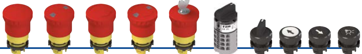
Przycisk awaryjny Ø 40 "wciśnij-pociągnij" Przycisk awaryjny Ø 40 "wciśnij-pociągnij" ze wskaźnikiem zadziałania Przycisk awaryjny Ø 40 "obróć aby zwolnić" Przycisk awaryjny Ø 40 "obróć aby zwolnić" ze wskaźnikiem zadziałania Przycisk awaryjny Ø 40 z kluczykiem Przełącznik krzywkowy, 2 lub 3 pozycyjny Przełącznik, 2 lub 3 pozycyjny Przycisk GÓRA Przycisk DÓŁ Przycisk OŚWIETLENIE
